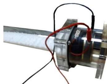
氣柱共鳴實驗
